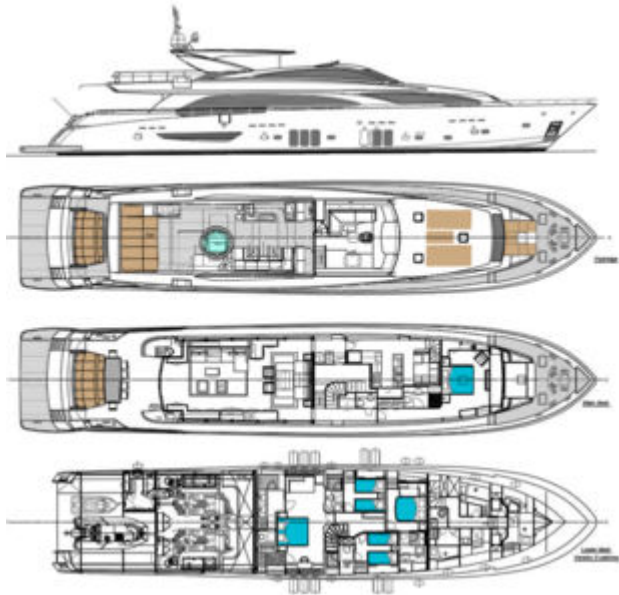
Layout ASCENSION - Couach 3700
